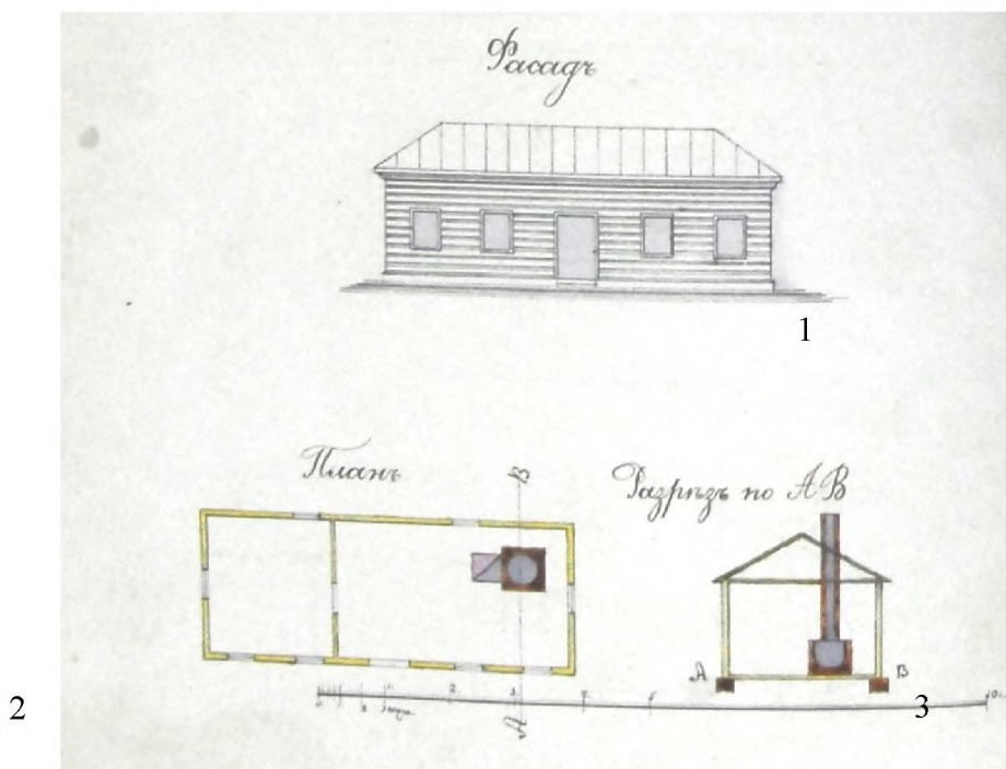
Рис. 1 – Проект мещанина И.П. Кричевцова на постройку здания для изготовления мыла: 1 – фасад здания; 2 – план проекта; 3 – здание на рисунке в разрезе
